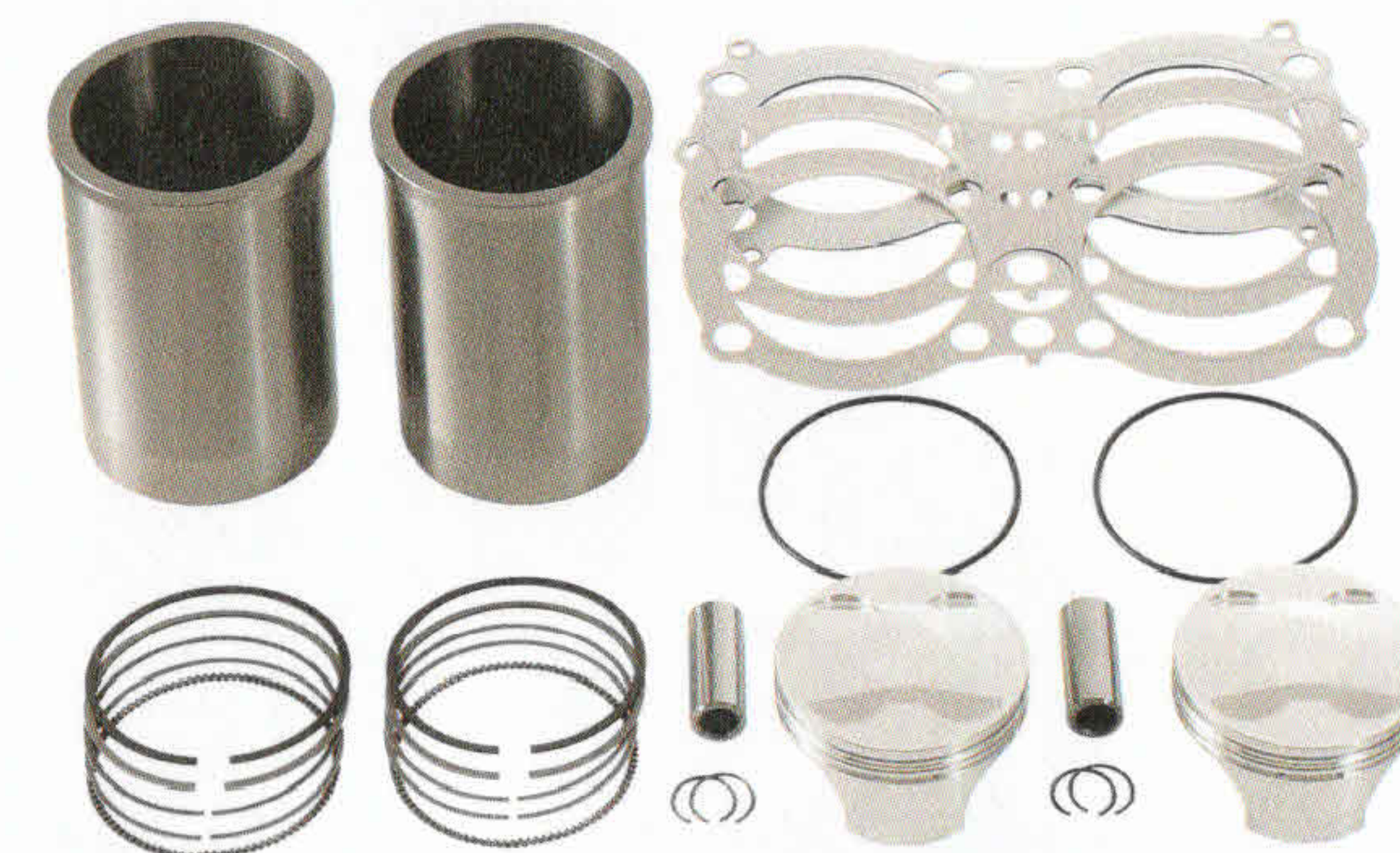
JB-POWER CP \phi 79 W650 (シリンダーライナー付) ¥98,000.- (税別)
