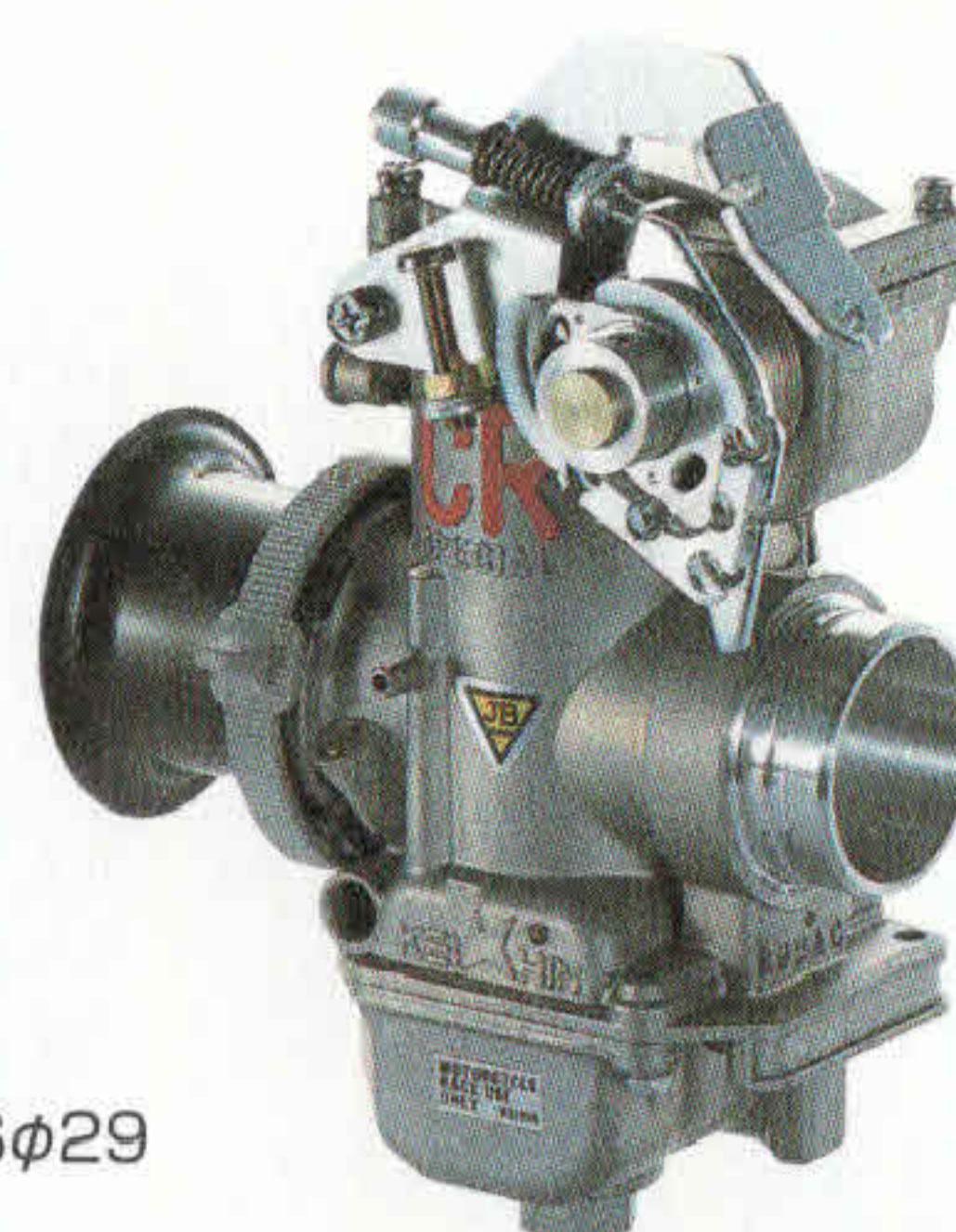
JB-POWER CRSφ38 SR400/500 ¥31,000.- (税別)
