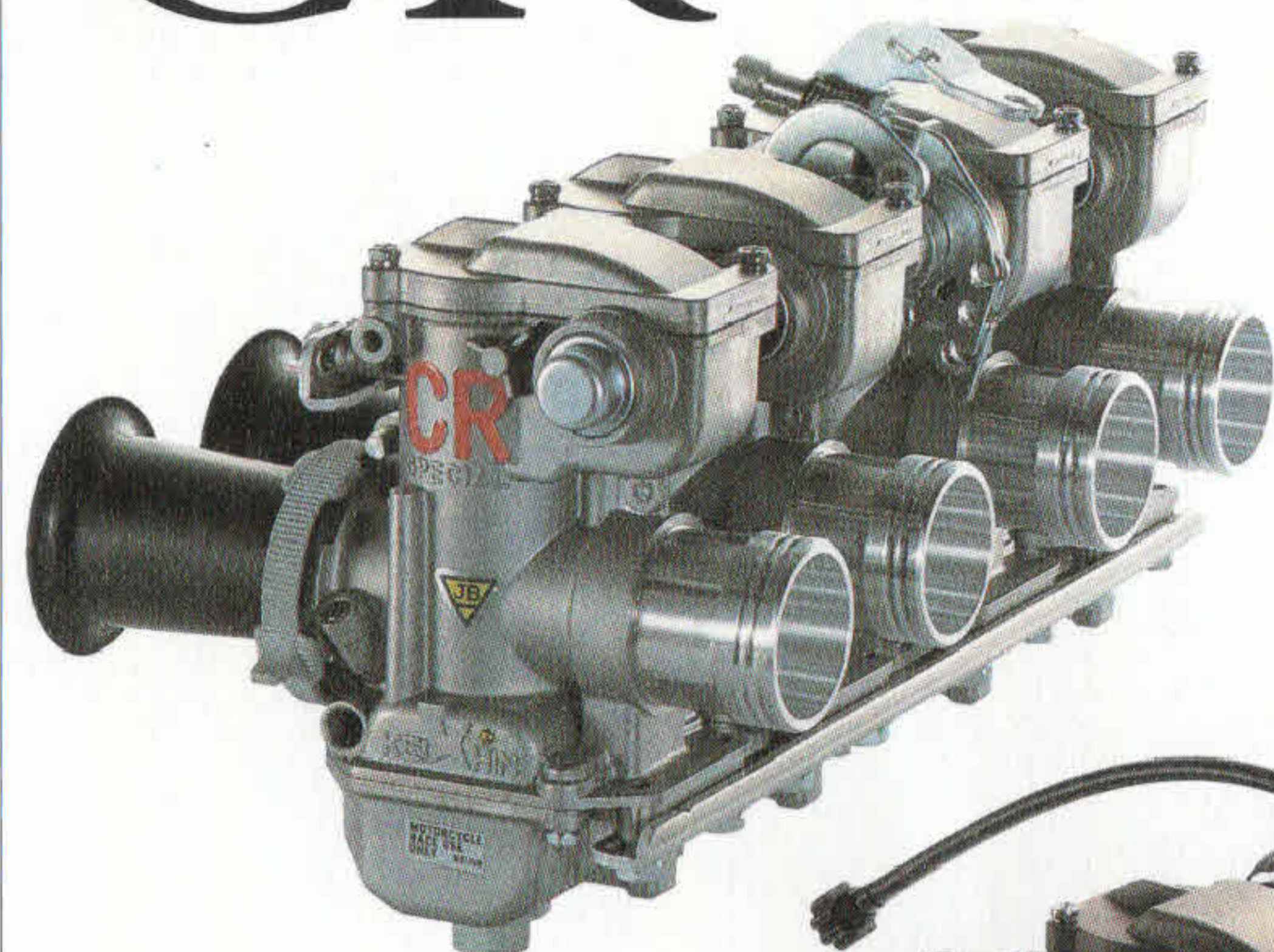
JB-POWER CRSφ29 CB750F ¥85,000.- (税別)
