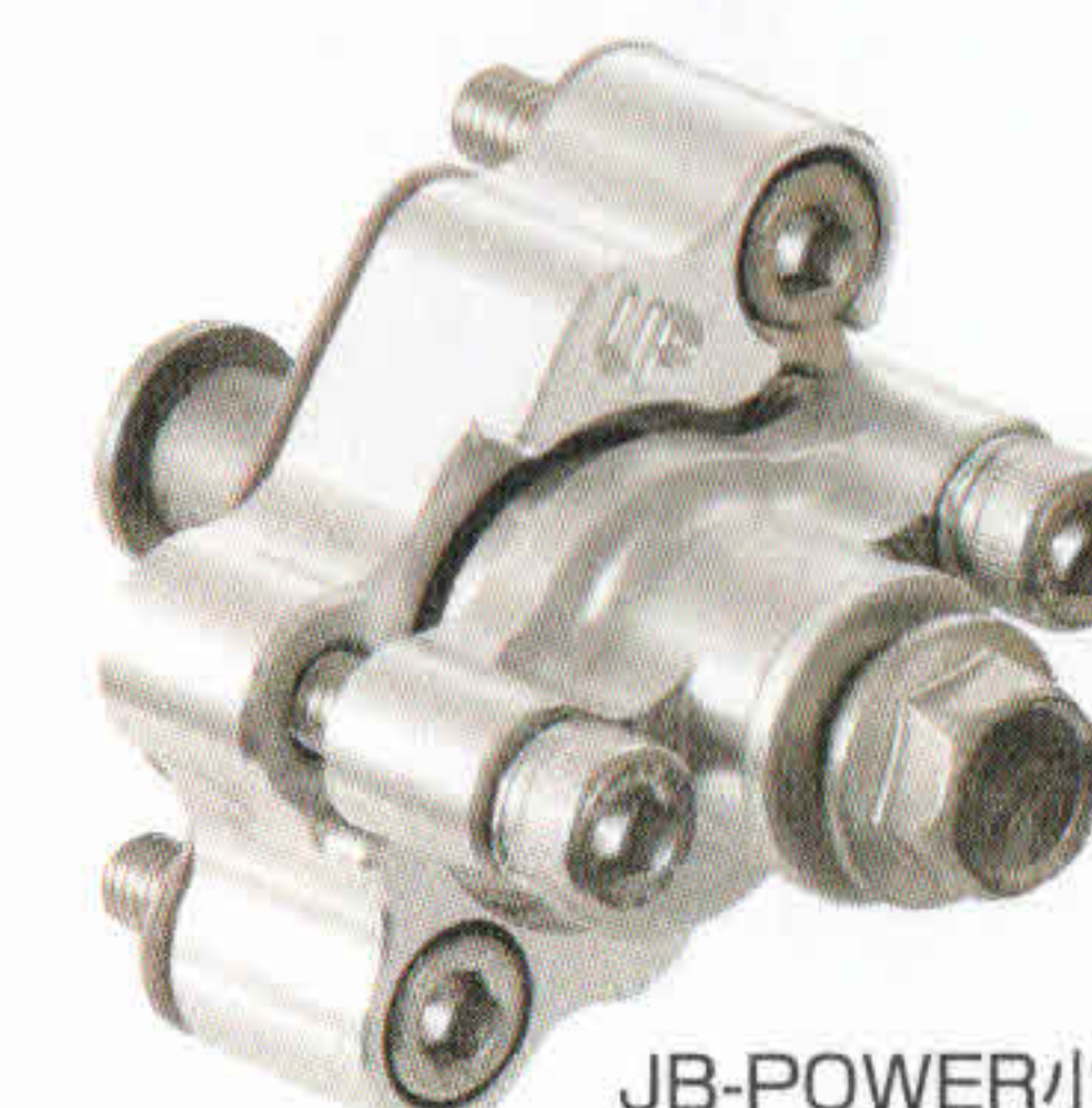
JB-POWER 小型オート カムチェーンテンショナー Z I / Z II ZEPHYR750- '00 ¥20,000.- (税別)
