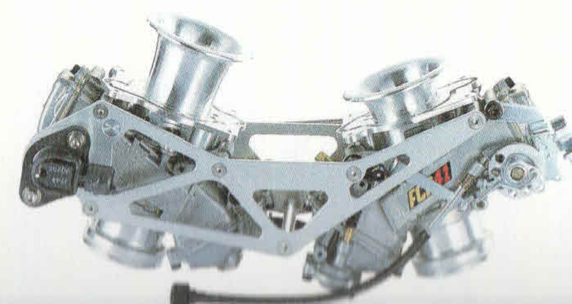
JB-POWER インテークマニホールドセット KZ1300 ¥90,000.- (税別)
